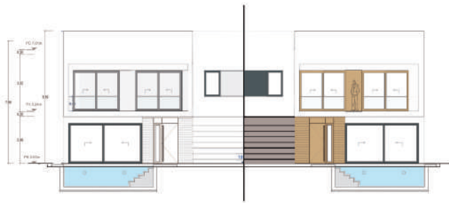
Alzado Oeste
